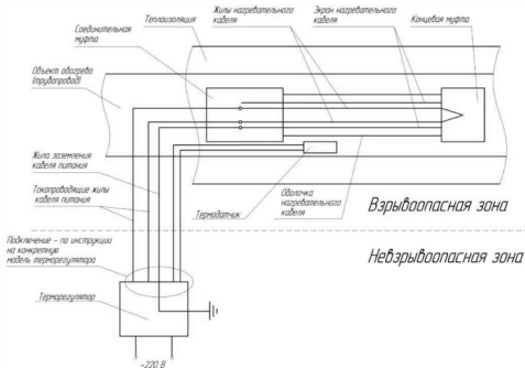
Рисунок 3. Схема монтажа нагревательной секции.
